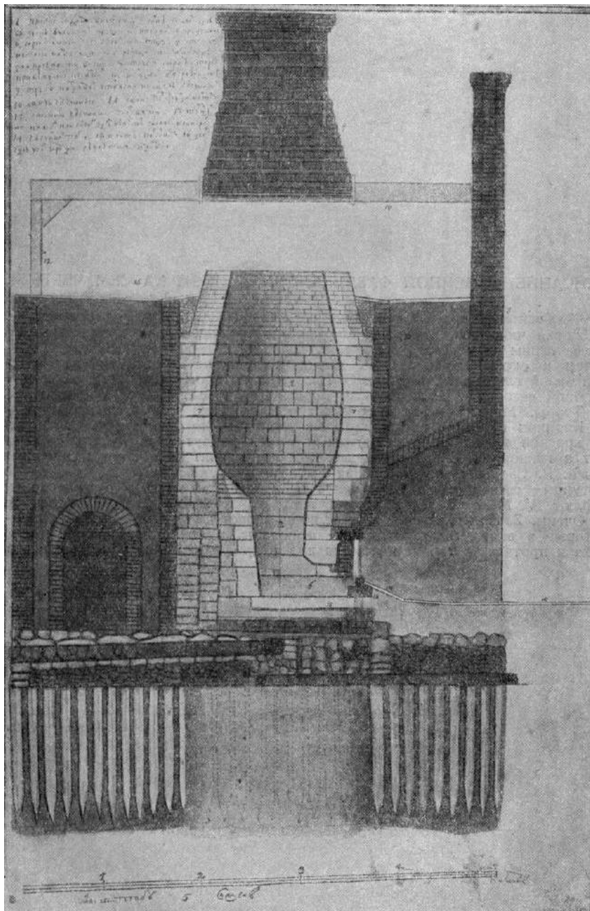
[ПРОФИЛЬ ДОМНЫ]
